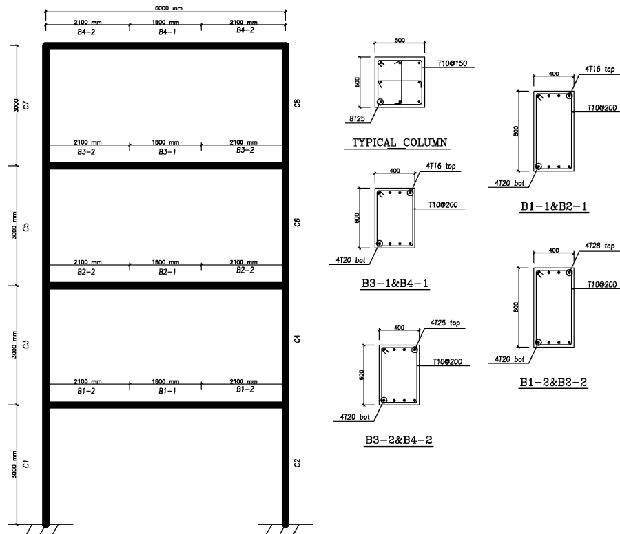
Frame Elevation
